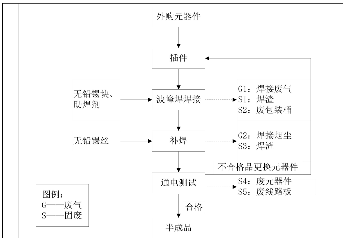
图 2-2 半成品生产线工艺流程及产污环节图
