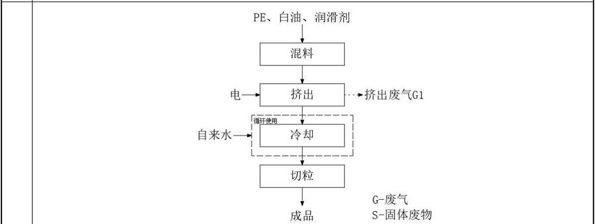
图 2.2-1 改性塑料制造工艺流程及产污环节图
